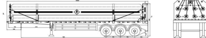
9管束式拖车参数 9 TUBES
