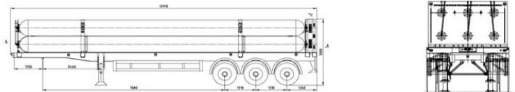
6管束式拖车参数 6 TUBES
